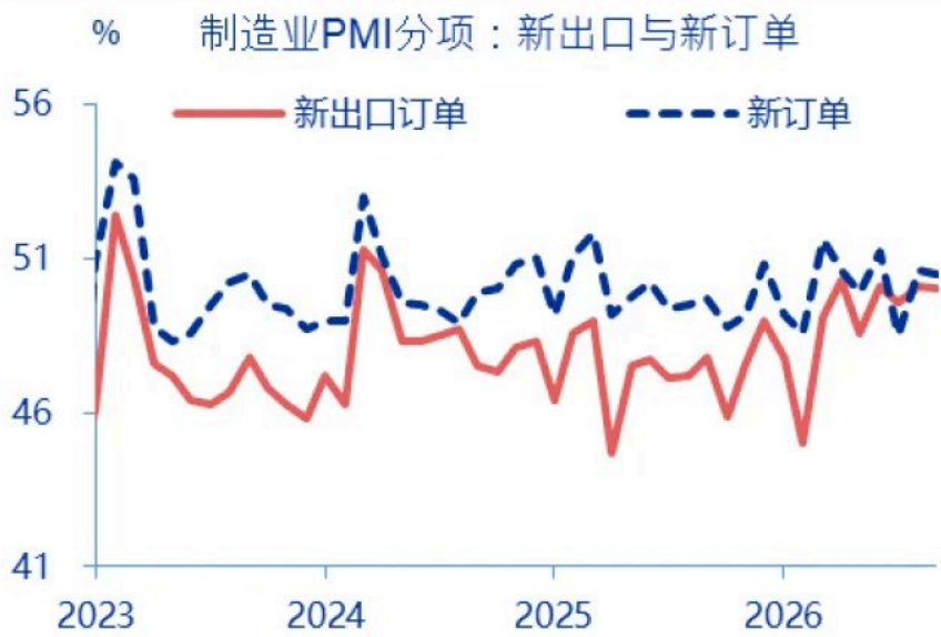
图 17：制造业 PMI 新出口订单、新订单分项
